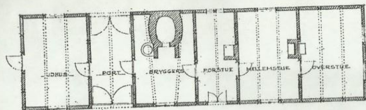
Hans Krogs rekonstruktion, sydfacade og grundplan (ca. 1:200).
